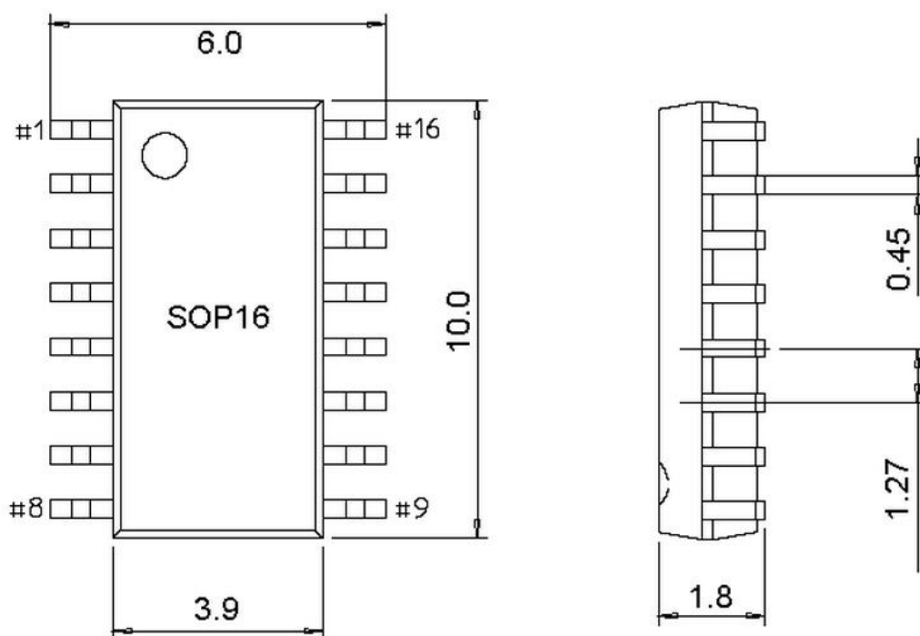
SOP16
