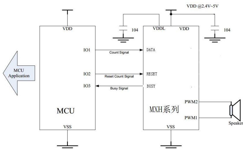
图 2：如下：2.4V 至 5V 电路参考
