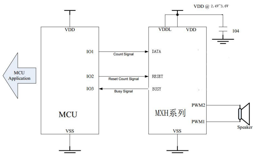
图 1：如下：2.4V 至 3.6V 电路参考
