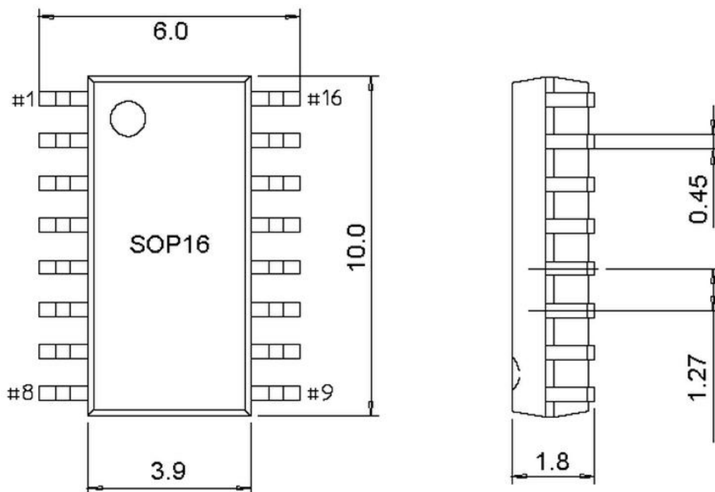
SOP16
